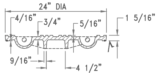
COVER SECTION N.T.S.
