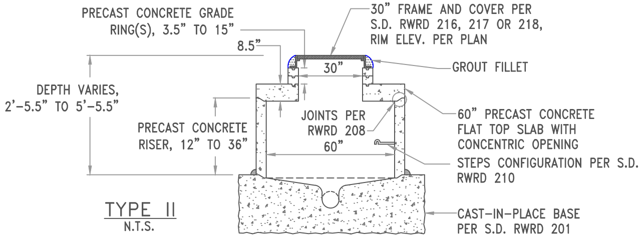
TYPE I N.T.S.
