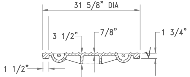
COVER SECTION N.T.S.
