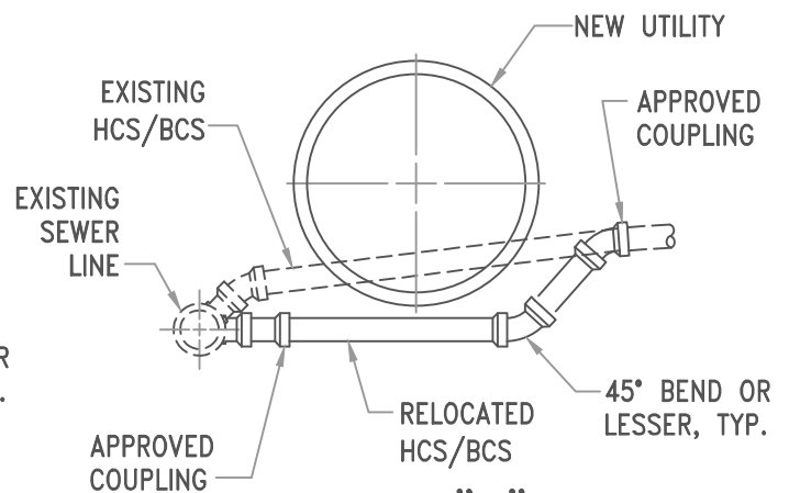
CASE "D" N.T.S.
