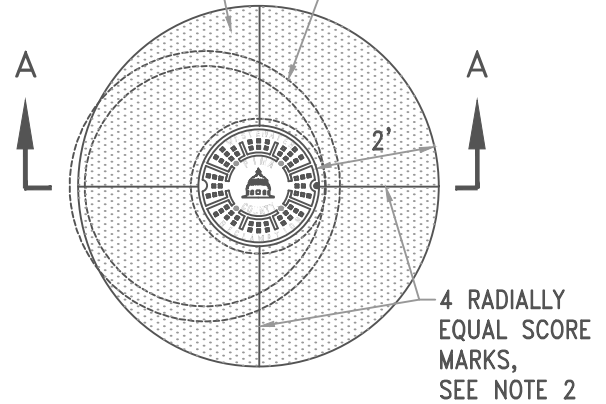
PLAN VIEW ROUND COLLAR N.T.S.
