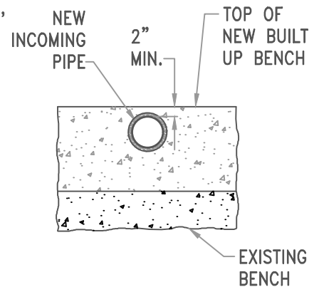
SECTION B-B N.T.S.
