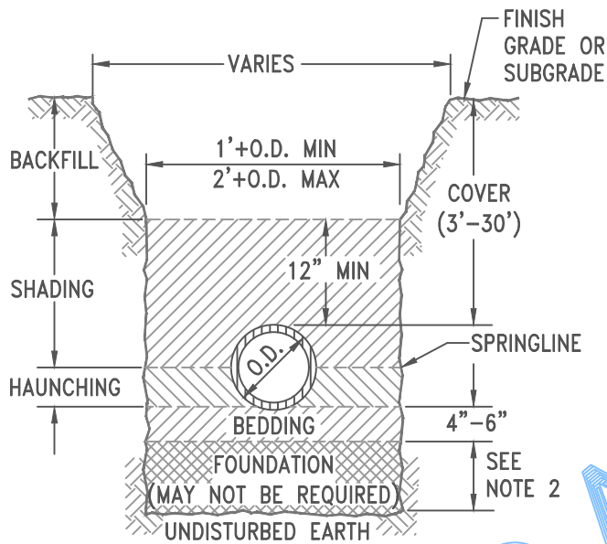
FLEXIBLE PIPE TRENCH DETAIL N.T.S.
