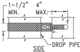
BRACKET DETAIL N.T.S
