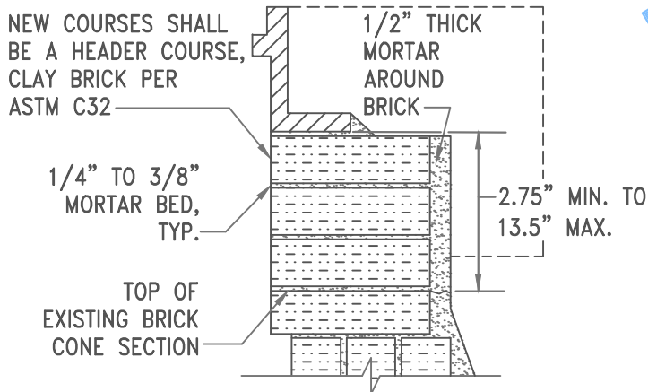
BRICK ADJUSTMENT N.T.S.
