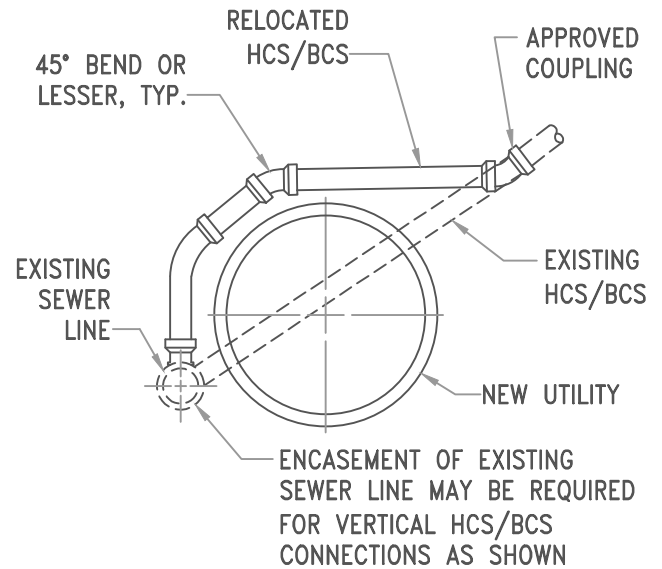
CASE "B" N.T.S.
