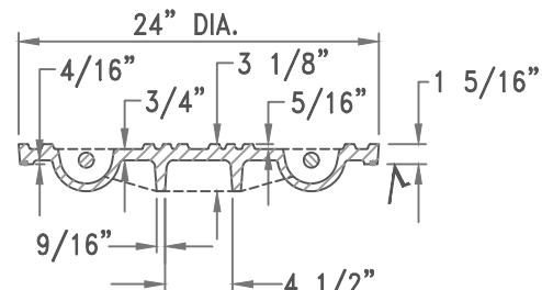
COVER SECTION N.T.S.
