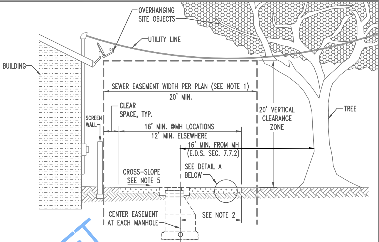
SECTION A-A (SEE DETAILS S.D. RWRD 109 & 110) N.T.S.
