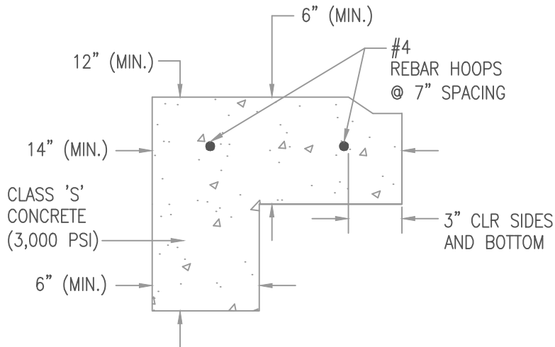
LEVELING COURSE DETAIL N.T.S.
