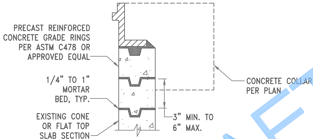
GRADE RING DETAIL N.T.S.
