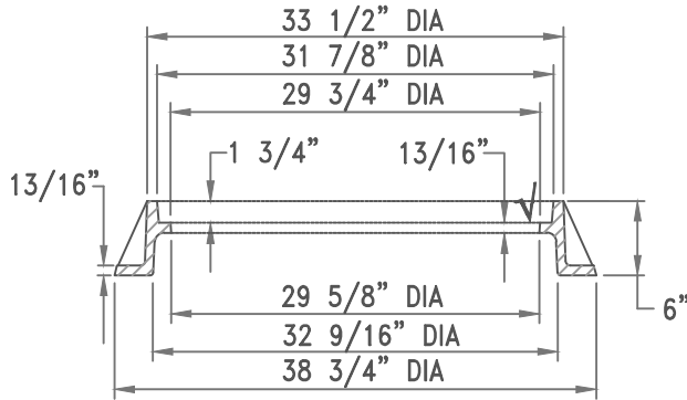
FRAME SECTION A-A N.T.S.
