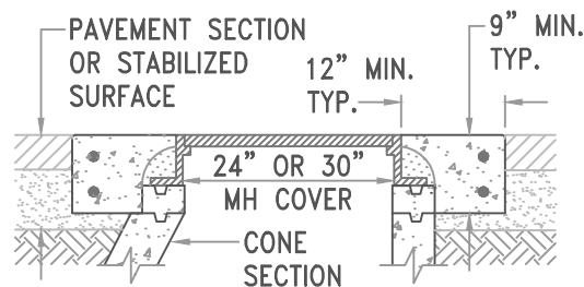
SECTION A-A FOR CONE-TOP N.T.S.
