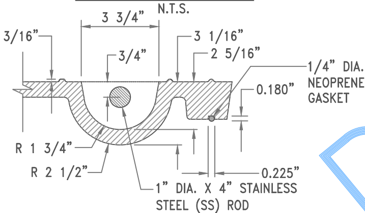
PICKBAR RECESS DETAIL N.T.S.
