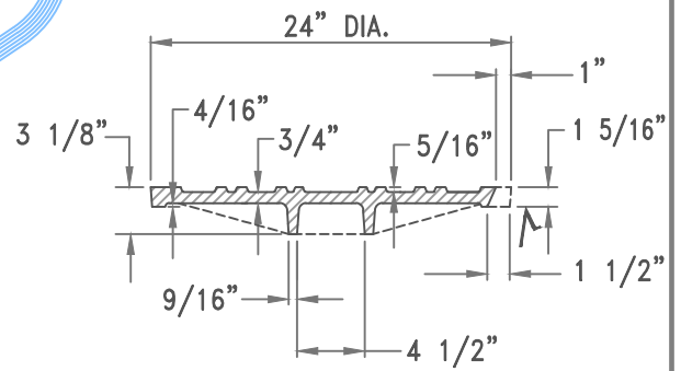
COVER SECTION N.T.S.
