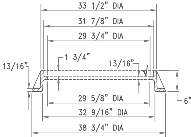
FRAME SECTION A-A N.T.S.
